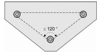
Bild 5: Prinzipskizze Winkeldefinition punktgelagerte VSG-Scheibe
